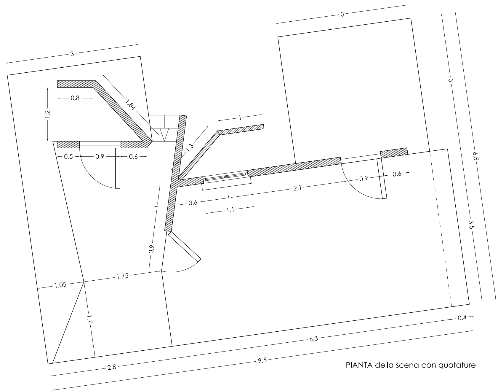
PIANTA della scena nella sala A - Teatro India
