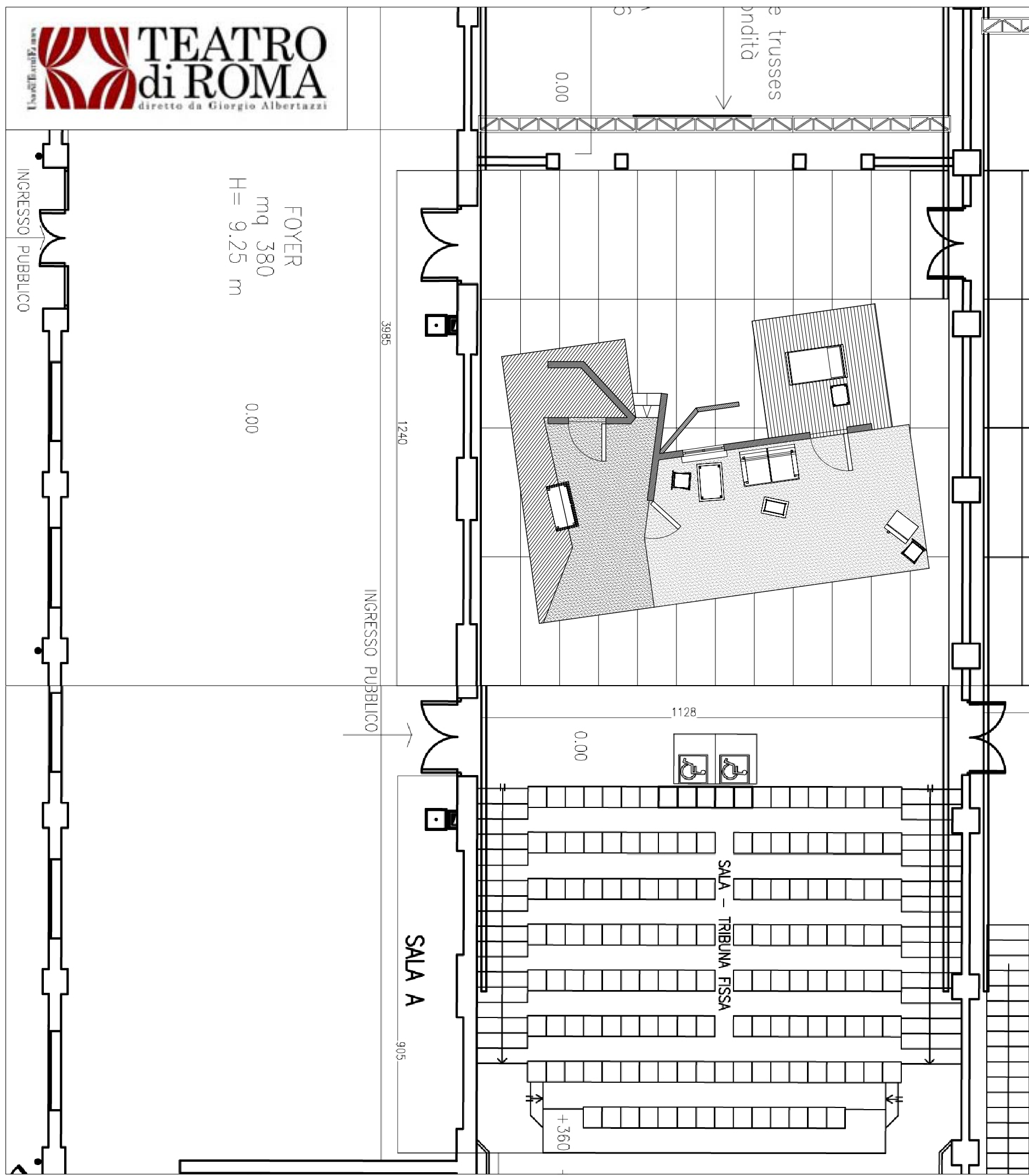
PIANTA della scena nella sala A - Teatro India
